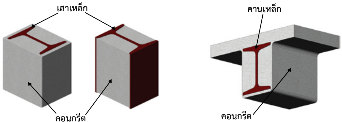
ก. การป้องกันโครงสร้างเหล็ก เสาและคานหน้าตัดรูปตัว I โดยการหุ้มด้วยคอนกรีต
